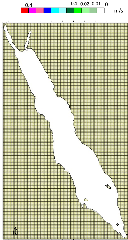
Tides (Abohadima & Rakha 2013)
